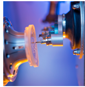
Glasgravur mit separater Werkzeugspitze.
