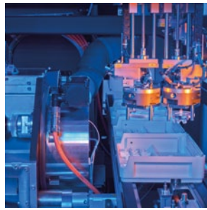
Las piezas de bloque se ordenan de nuevo en la bandeja de trabajo después del desbloqueo
